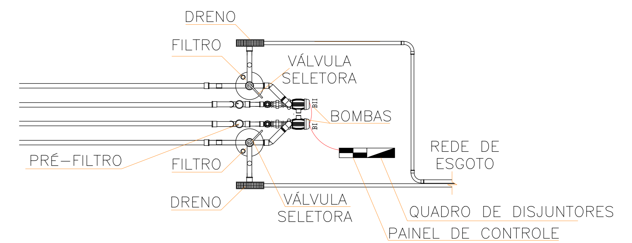
PLANTA BAIXA DE INSTALAÇÕES HIDRÁULICA DA PISCINA ADULTA unidades em metros esc: 1:100
