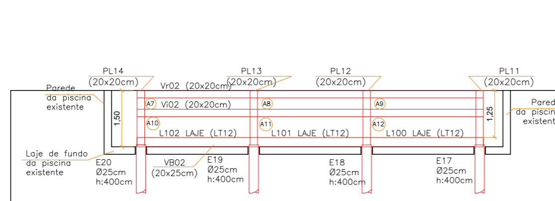
CORTE CC DE TODA A INFRAESTRUTURA E SUPERESTRUTURA TRECHO MAIS RASO DA PISCINA unidades em metros esc: 1:100
