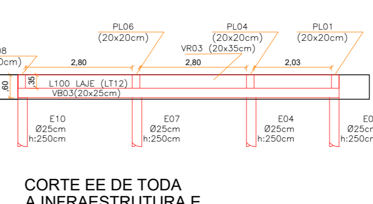
CORTE EE DE TODA A INFRAESTRUTURA E SUPERESTRUTURA TRECHO DA PISCINA INFANTIL unidades em metros esc: 1:100
