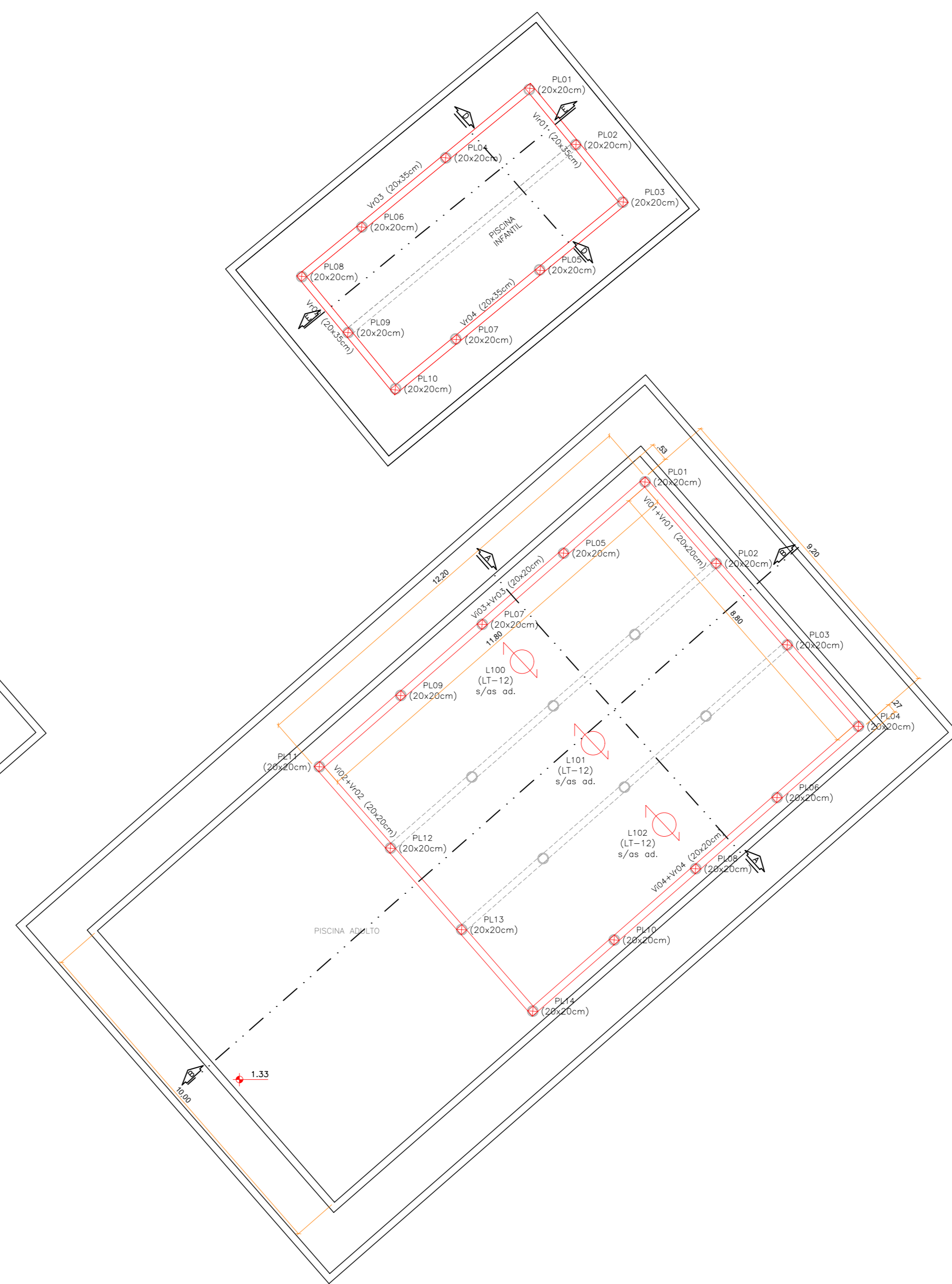
PLANTA BAIXA DE RECONSTRUÇÃO DA PISCINA ADULTA - PLANTA DE LOCAÇÃO DOS PILARES, VIGAS INTERMEDIÁRIAS E DE RESPALDO unidades em metros esc: 1:100
