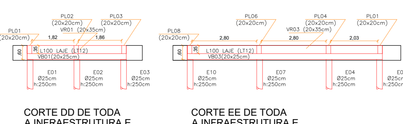
CORTE DD DE TODA A INFRAESTRUTURA E SUPERESTRUTURA TRECHO DA PISCINA INFANTIL unidades em metros esc: 1:100
