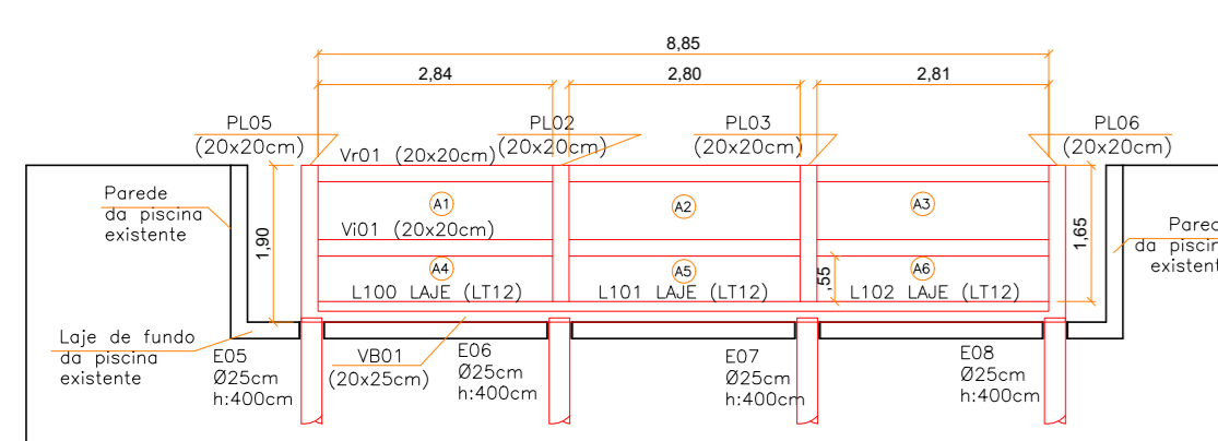
CORTE AA DE TODA A INFRAESTRUTURA E SUPERESTRUTURA TRECHO MAIS FUNDO DA PISCINA unidades em metros esc: 1:100
