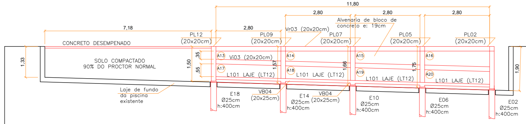
CORTE BB DE TODA A INFRAESTRUTURA E SUPERESTRUTURA - LATERAIS DA PISCINA unidades em metros esc: 1:100
