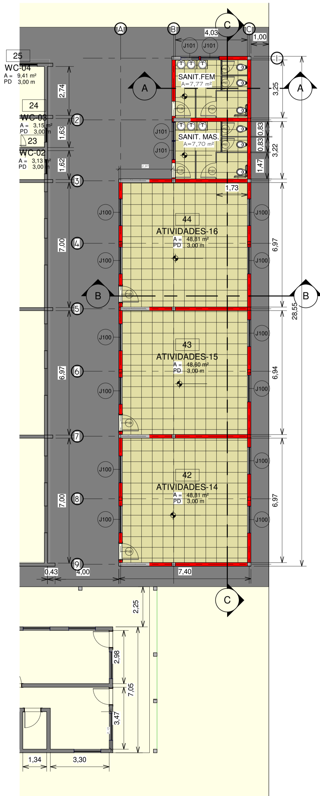
1 PAVTO. TERREO AMPLIAR 1 : 110
