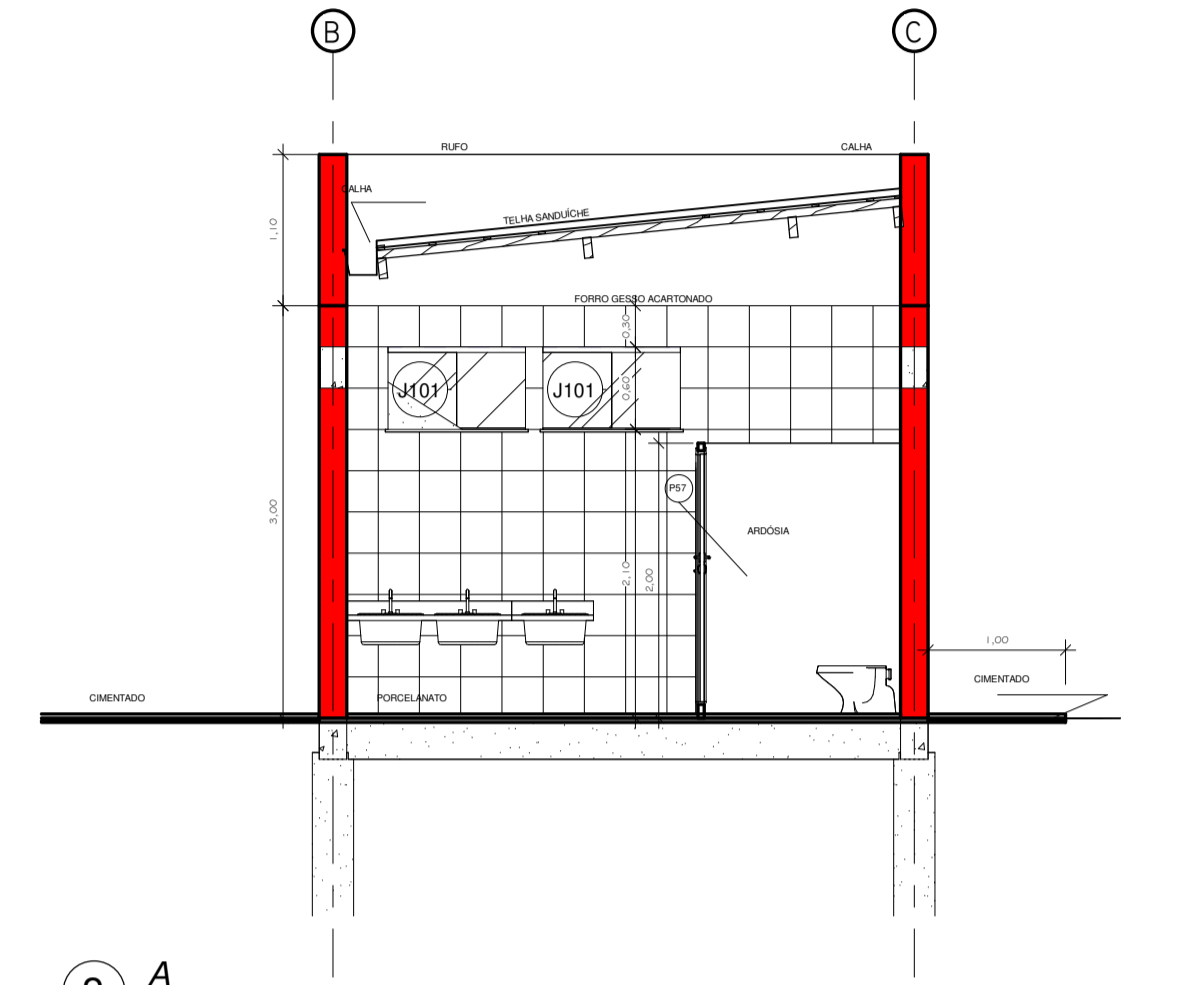
2 A 1 : 50
