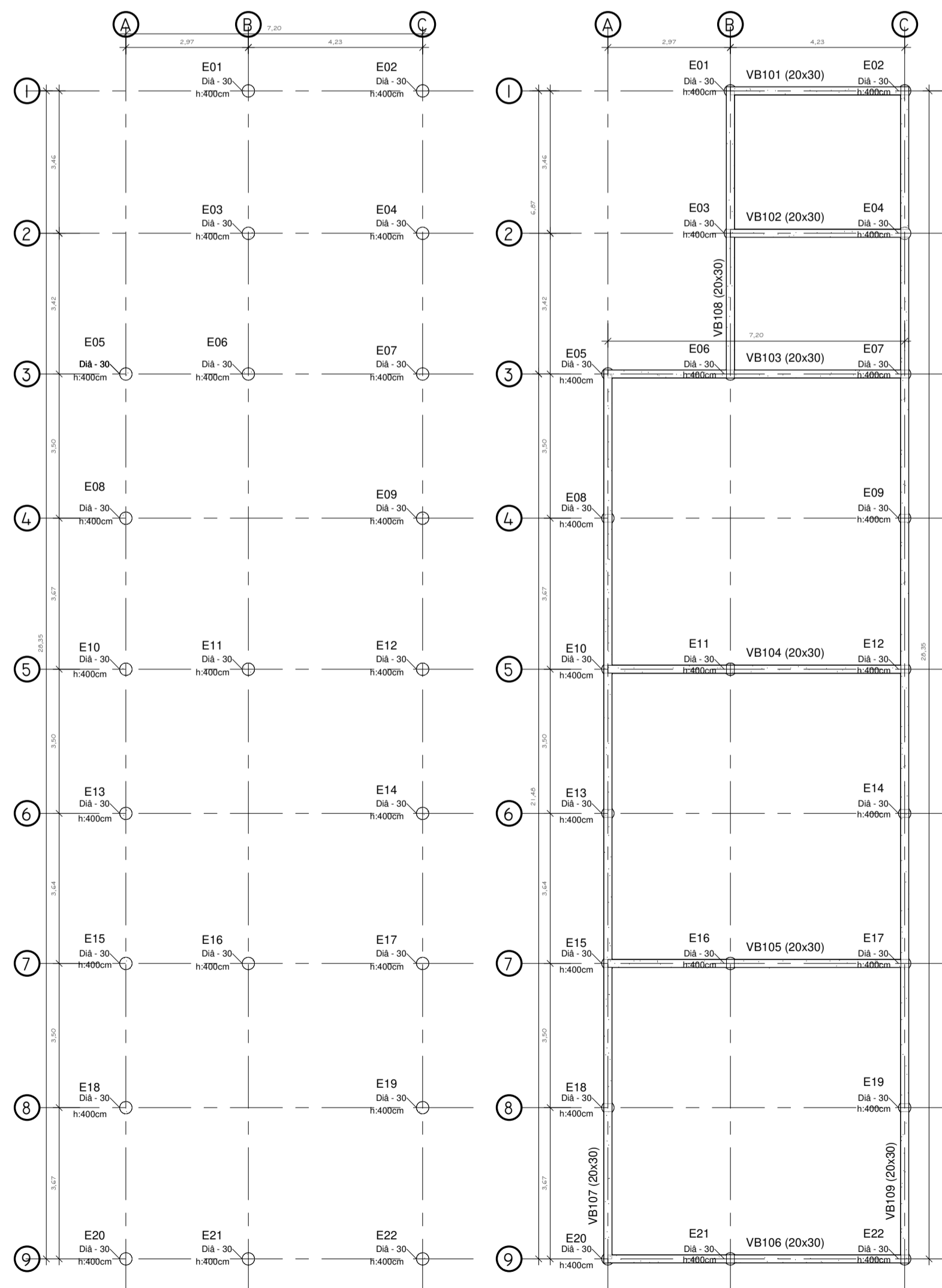
1 PLANTA DE LOCAÇÃO DAS ESTACAS 1 : 100
