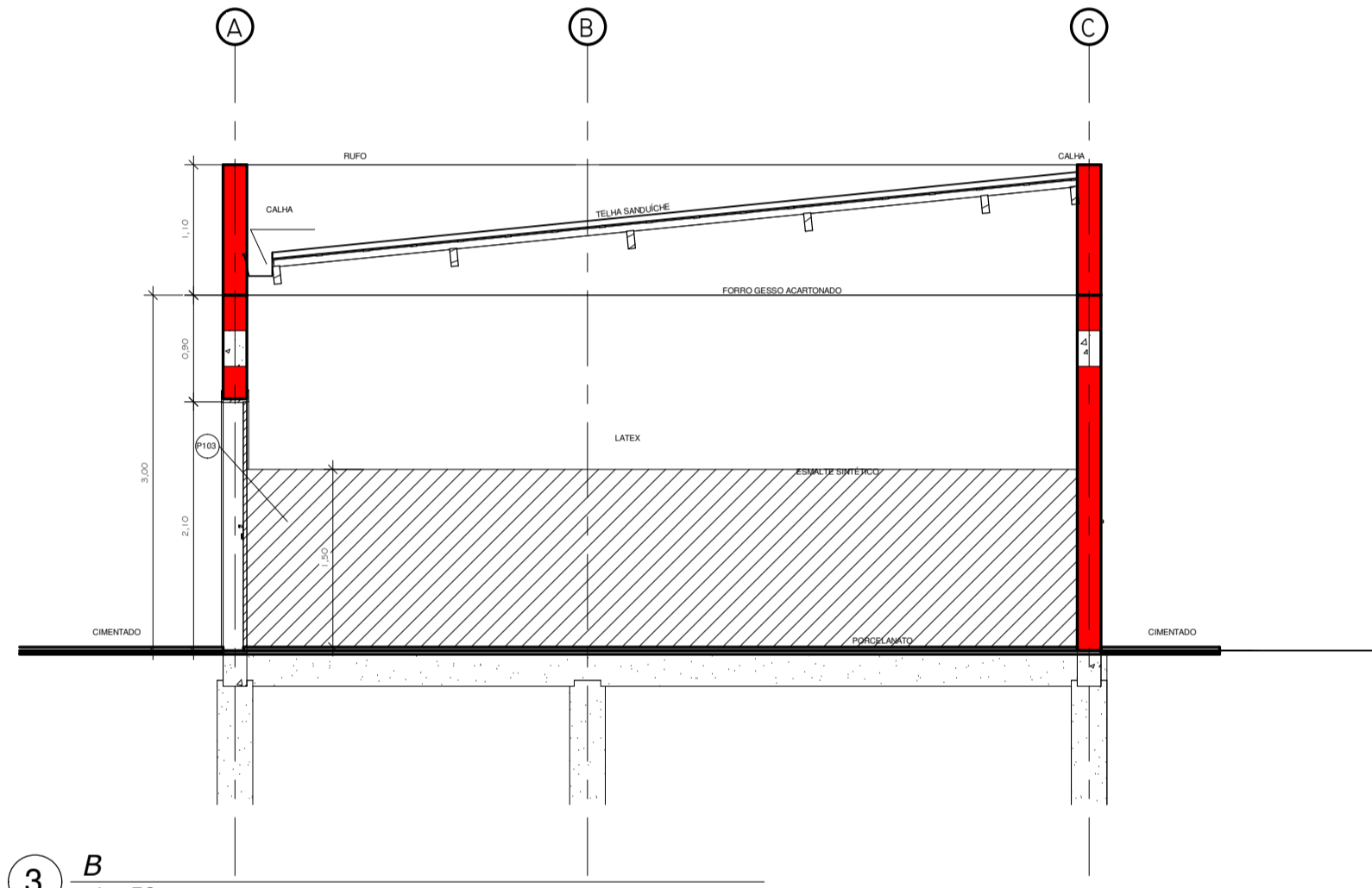
3 B 1 : 50
