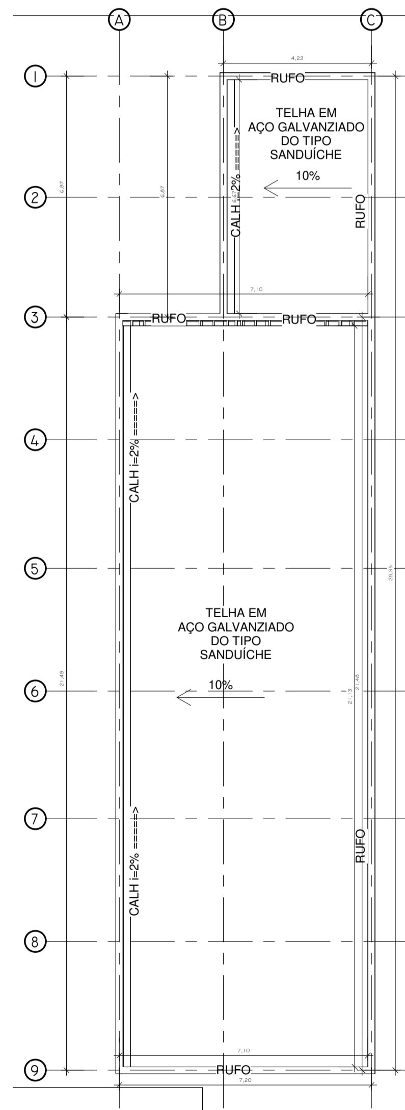
7 COBERTURA 1 : 100
