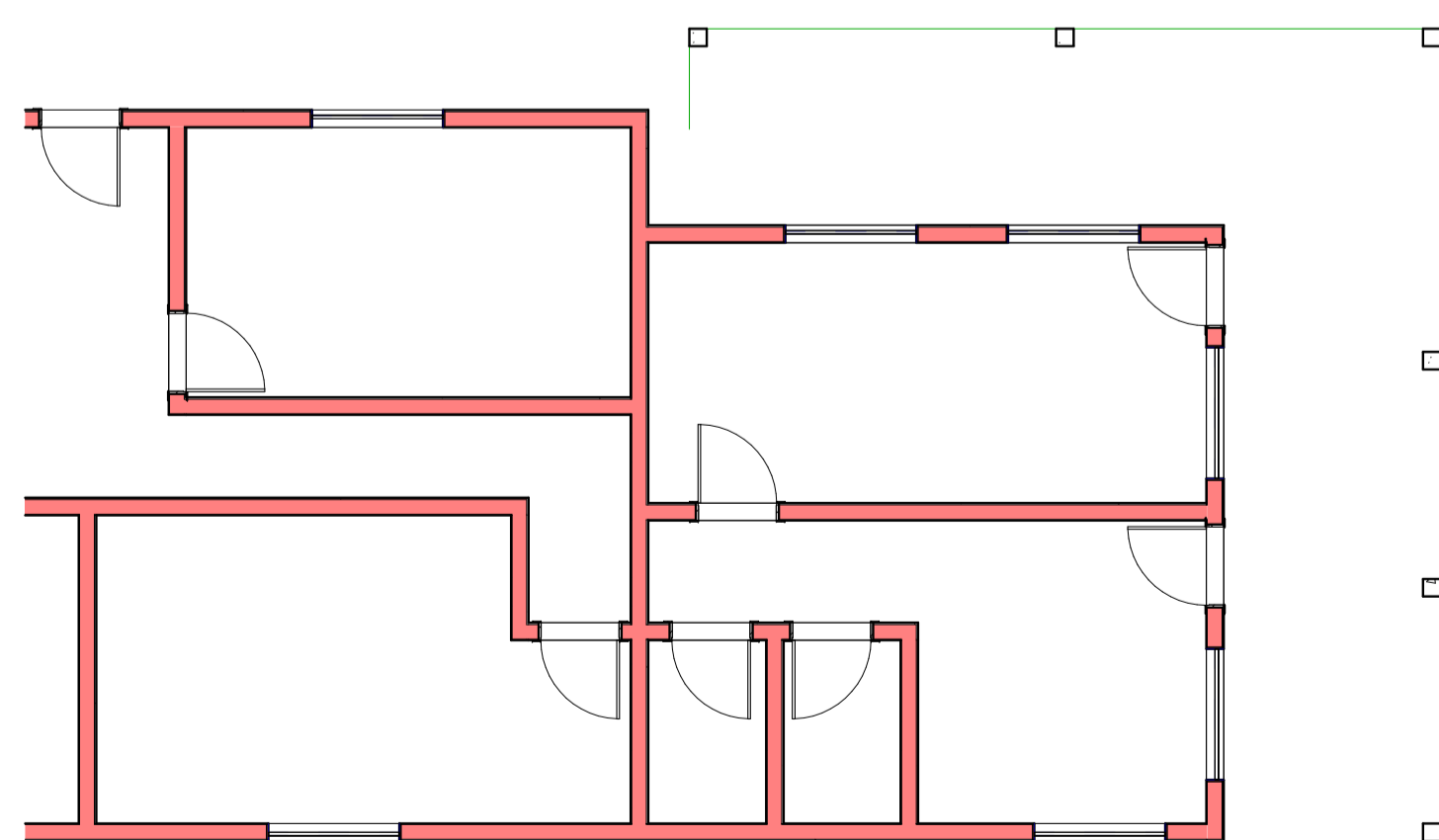
1 PROJETO ELÉTRICO 1 : 110
