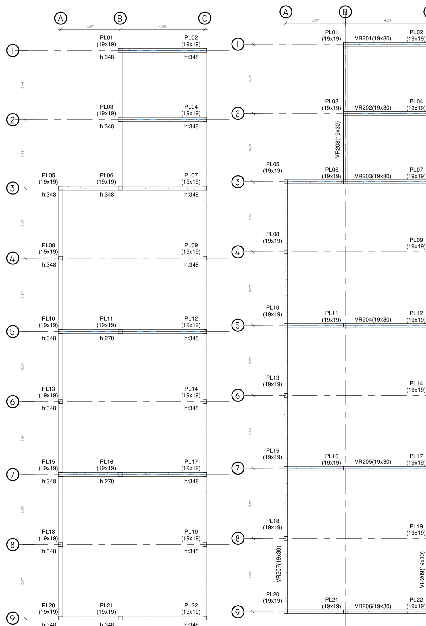
3 PLANTA DE LOCAÇÃO DOS PILARES 1 : 100
