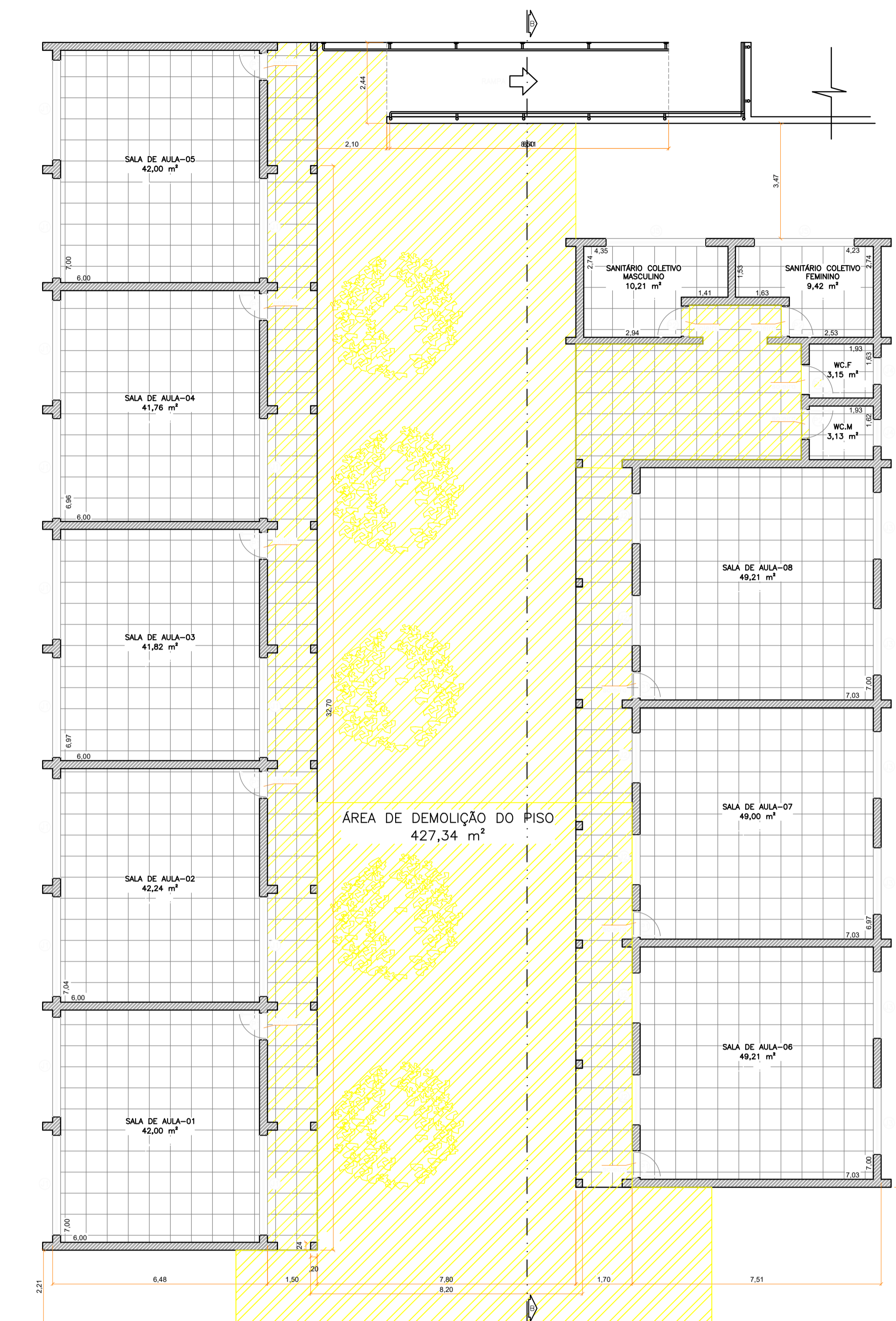
PLANTA BAIXA SITUAÇÃO ATUAL
