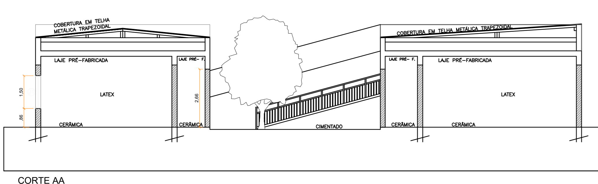
CORTE AA SITUAÇÃO ATUAL
