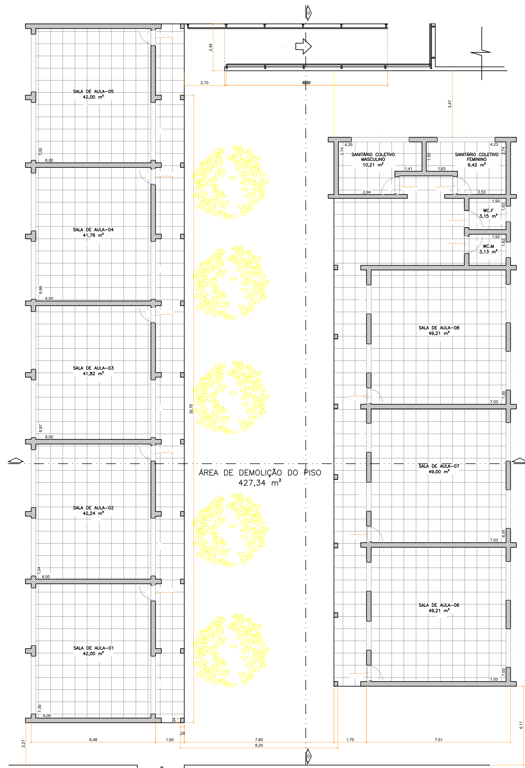
PLANTA BAIXA SITUAÇÃO ATUAL
