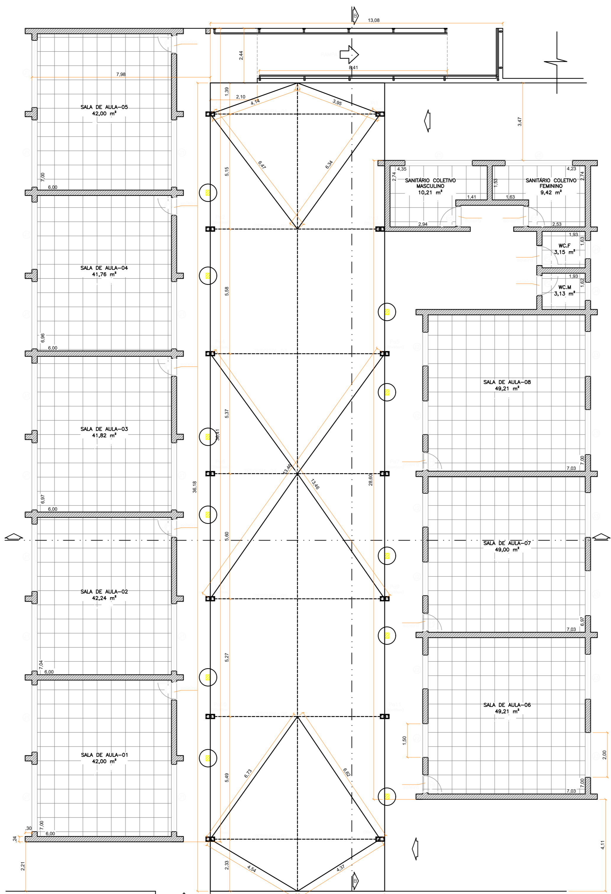
PLANTA BAIXA SITUAÇÃO PRETENDIDA
