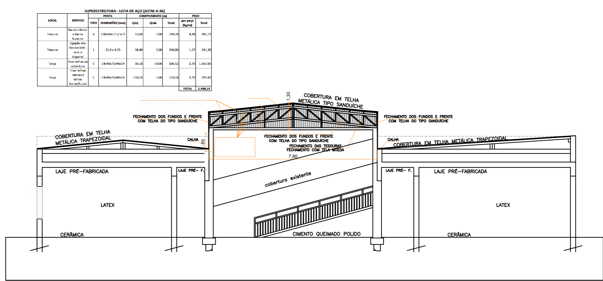
CORTE AA SITUAÇÃO PRETENDIDA TESSOURA POSICIONADA AOS FUNDOS DA EDIFICAÇÃO
