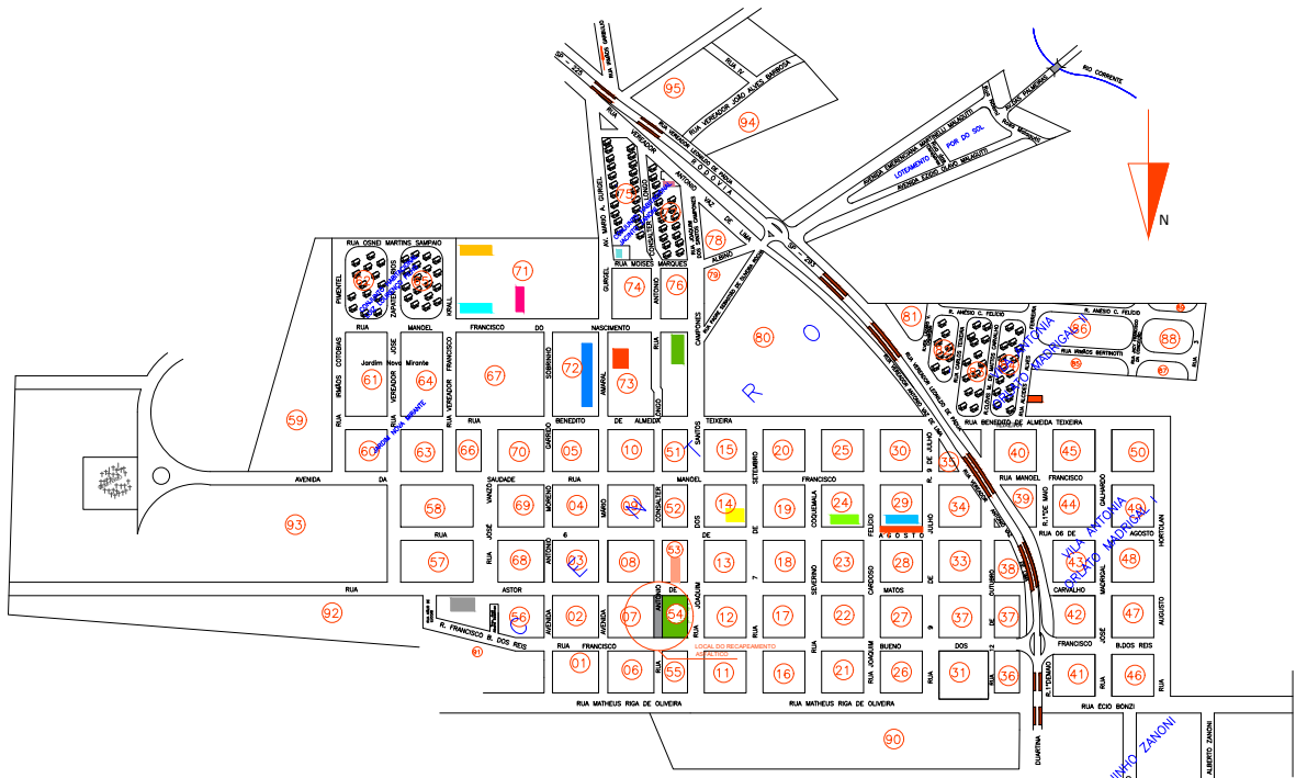
PLANTA DE LOCALIZAÇÃO DO RECAPEAMENTO ASFÁLTICO A = 640.00 M 2
