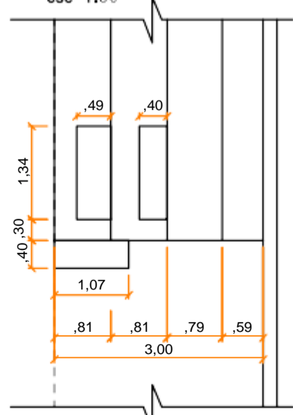
PLANTA BAIXA - Situação Atual Dimensões da Escada unidades em metros esc 1:50
