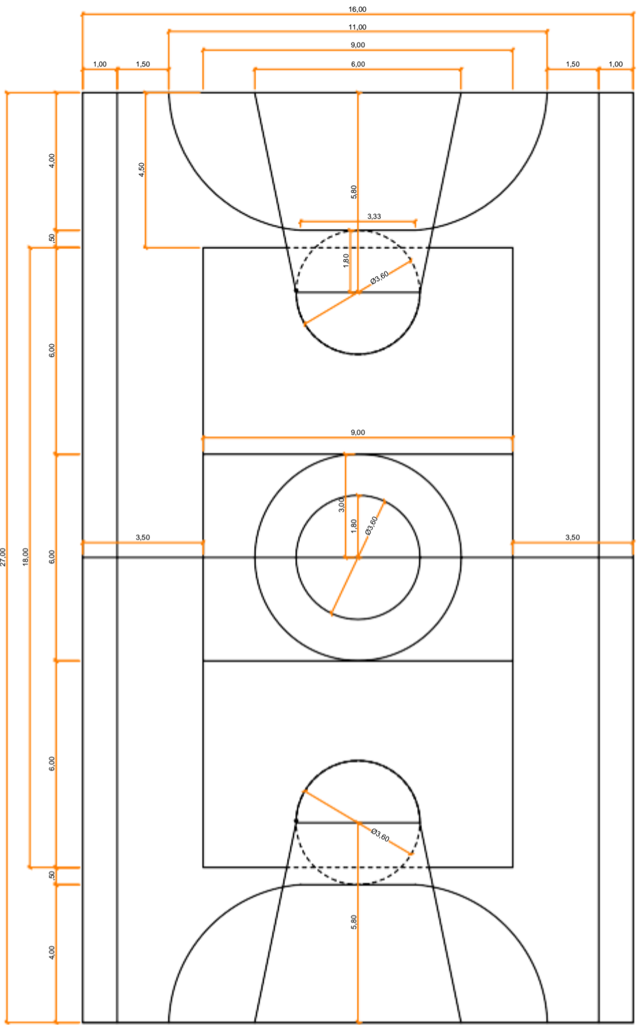
DETALHE DA DEMARCAÇÃO DA QUADRA POLIESPORTIVA unidades em metros esc 1:100
