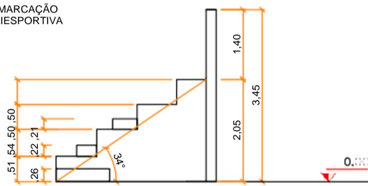
CORTE AA - Situação Atual Dimensões da Escada unidades em metros esc 1:50
