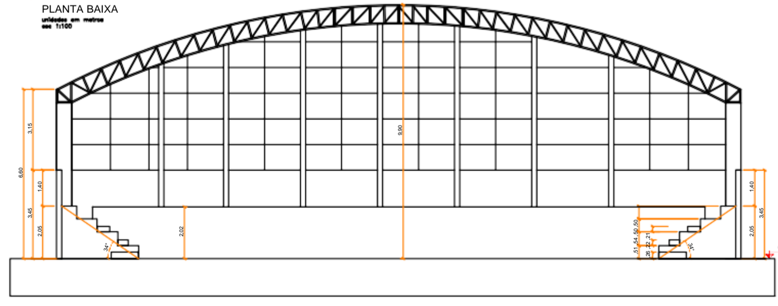
CORTE AA unidades em metros esc 1:50
